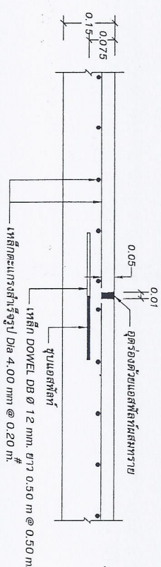
LONGITUDINAL JOINT มาตราส่วน No Scale
